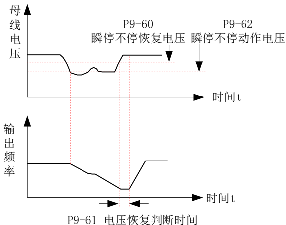
图 7-28 瞬停不停过程示意图
