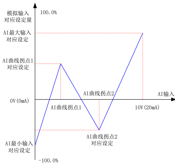
图 7-14 AI 曲线 4 和曲线 5 的设定
