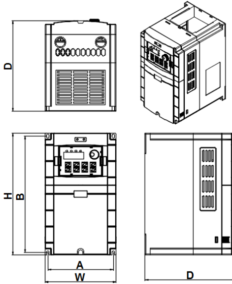
图 2-1 变频器外壳尺寸
