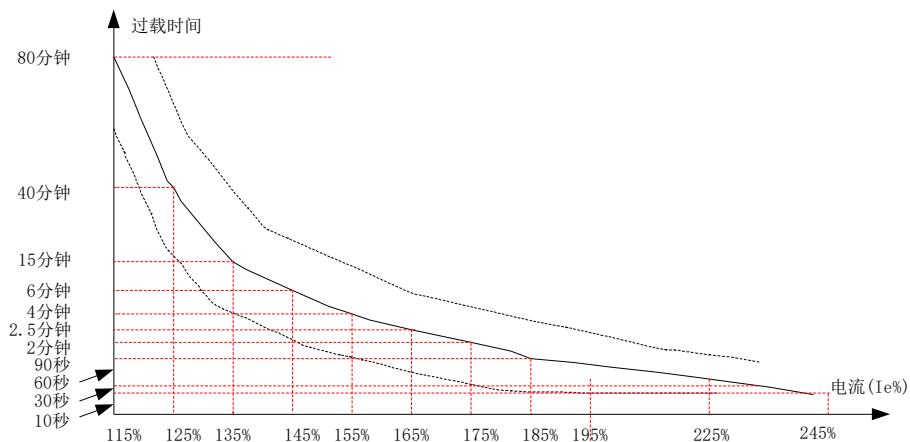
图 7-27 电机过载保护反时限曲线示意图
