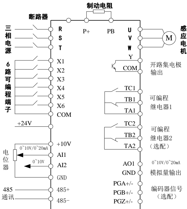
图 4-1 基本运行配线图
