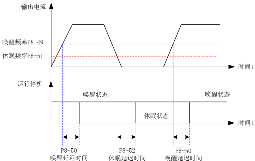
图 7-26 休眠与唤醒功能设置
