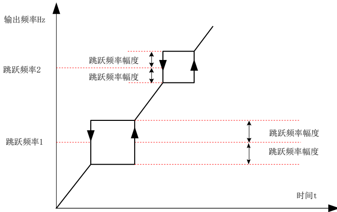
图 7-20 跳跃频率及范围示意图
